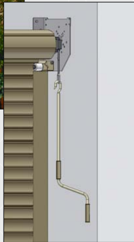
Nothandbedienung*
